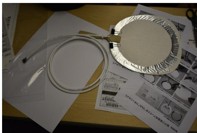
写真 3：自作アンテナの完成品
